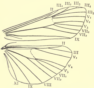
FIG. 272.—Wings of Nomophila noctuella .
