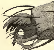
FIG. 43.—Foot of Epeira.
