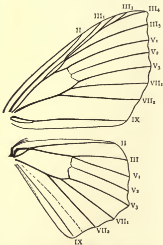
FIG. 341.—Wings of Synelys enucleata .
