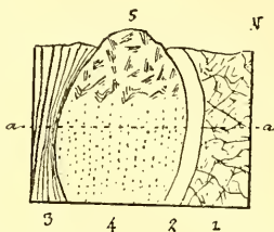
1. Roca cristalina descompuesta.—2. Pizarra carbonosa del culm.—3. Pizarras diversas del culm, trastornadas.—4. Pirita.—5. Coronamiento de limonita.
