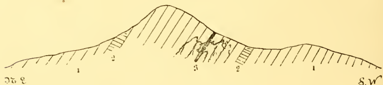
1. Caliza del eocénico medio metamorfozada.—2. La misma convertida en mármol.—3. Filón de magnetita y sus ramificaciones.
