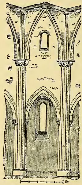
Fig. 361.—System of S. Andrea at Vercelli.
