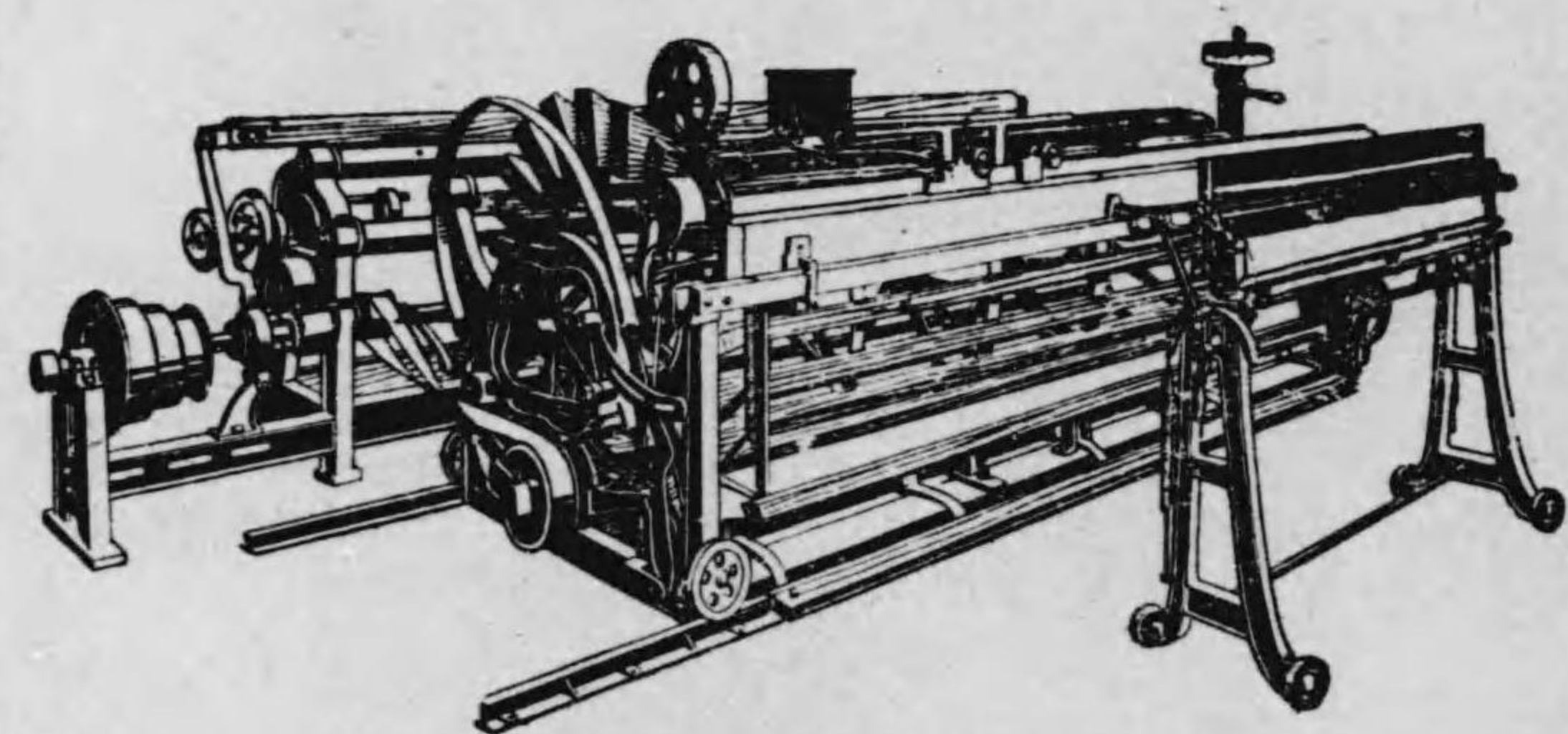
江口式S型分部整經機
