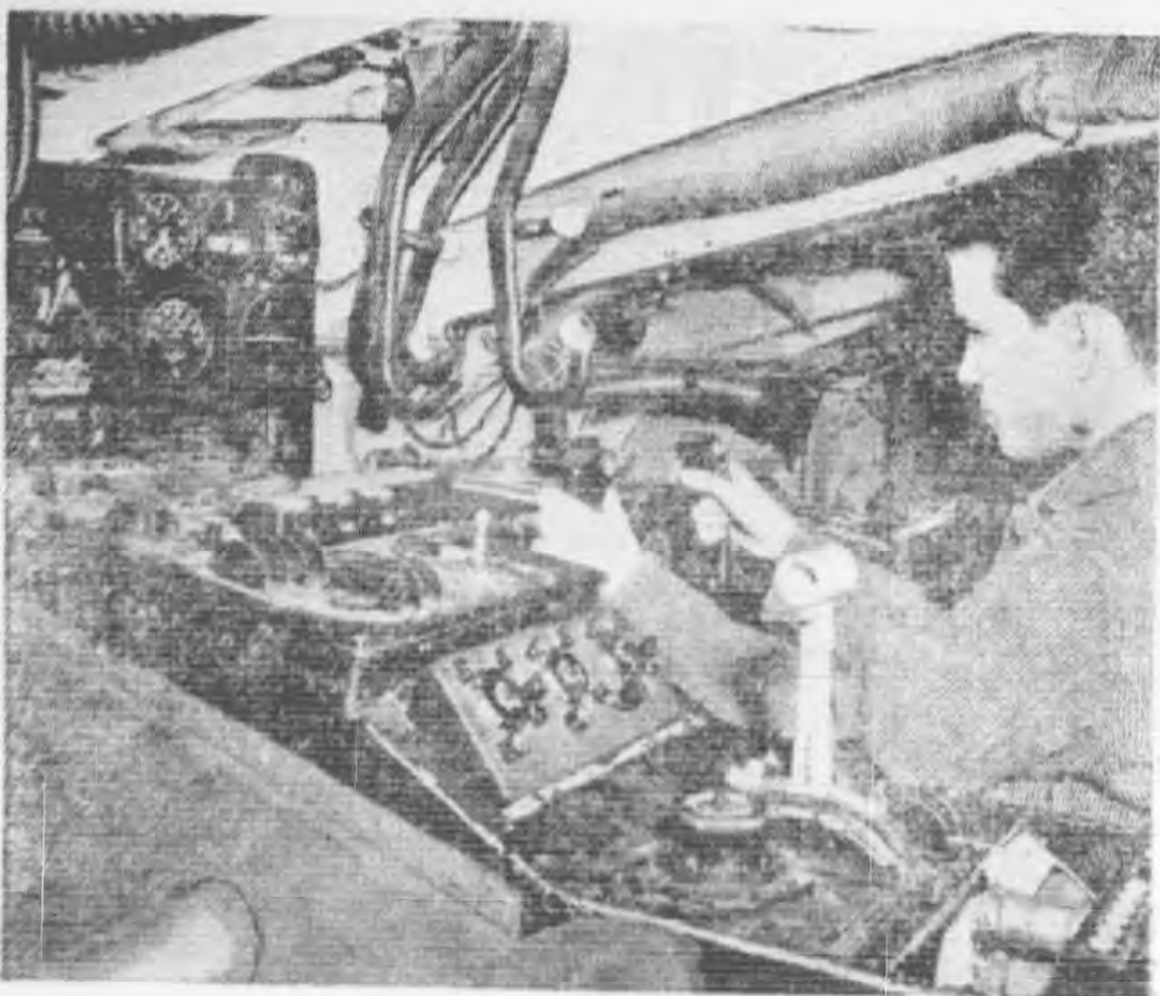
正機師的駕駛座（後左），機尾鎗手（後右）和領航員的座位（前）。正機師在駕駛座上的視線可以達任何角度。
