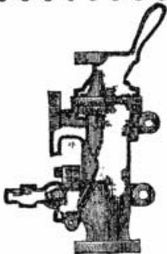
Универс. Инжекторъ
