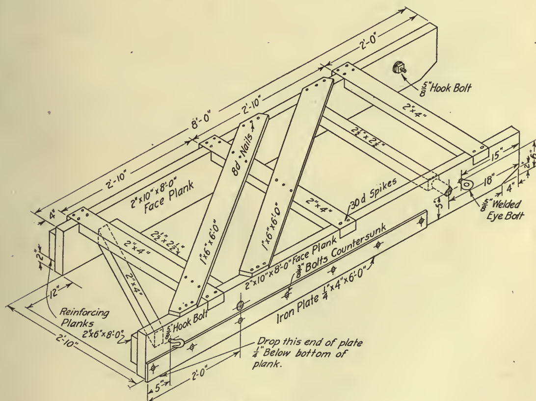
FIG. 79.—Road drag.
