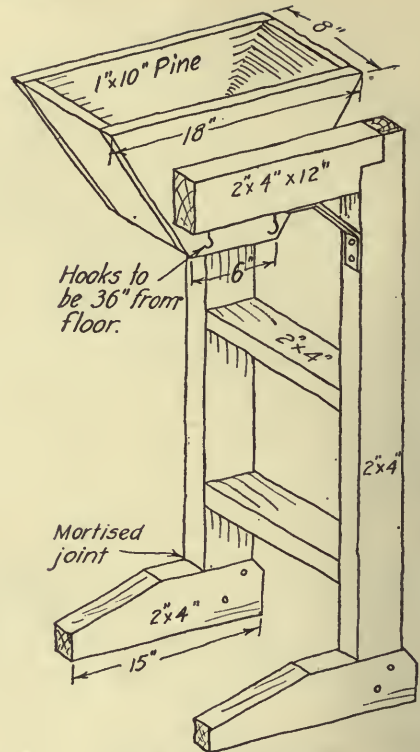
FIG. 76.—Sack holder.
