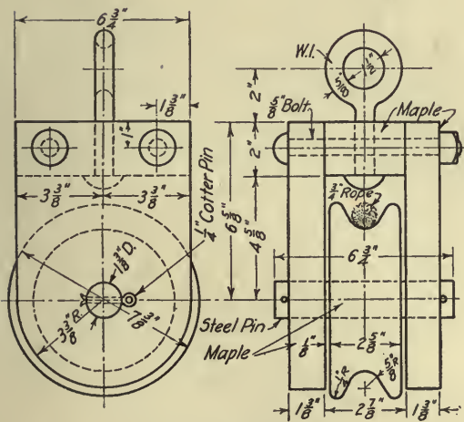
FIG. 90.—Sheave.
