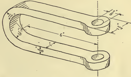
FIG. 72.—Clevis.
