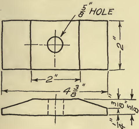
FIG. 161.—Button.
