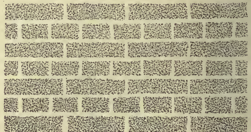
FIG. 107.—English bond.
