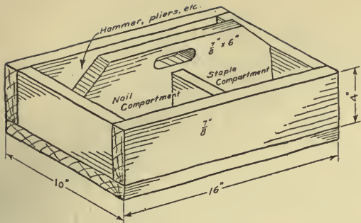
FIG. 70.—Tool box.
