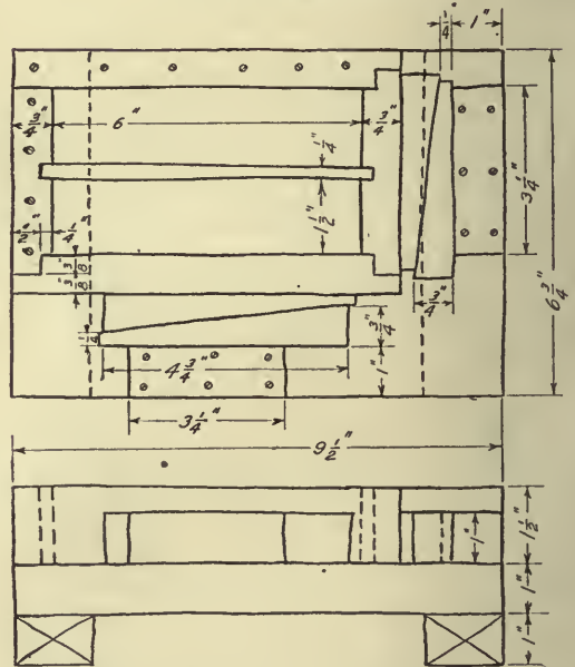
FIG. 76.—Sack holder.
