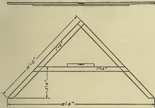
FIG. 172.—"A" frame.
