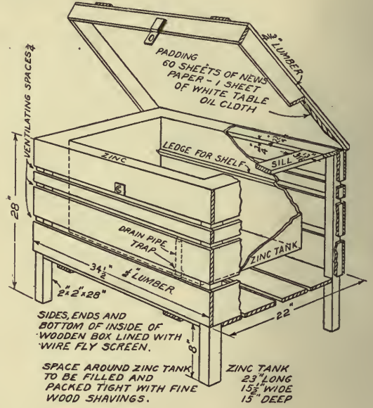
FIG. 87.—Ice box.
