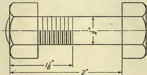
FIG. 59.—Dimensioned bolt.
