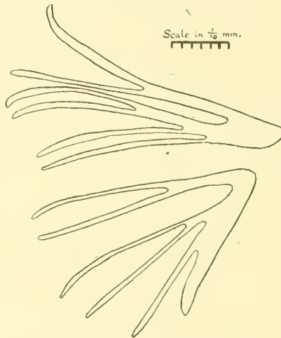
Orneodes microscopica .
