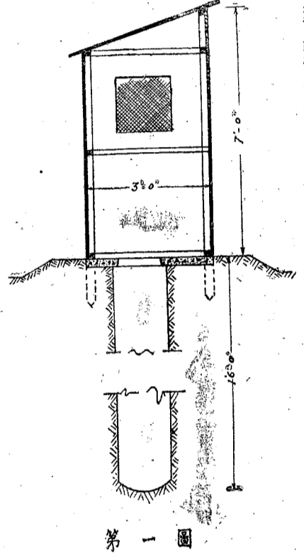
第一圖 爪哇式廁所建築法及使用原理
