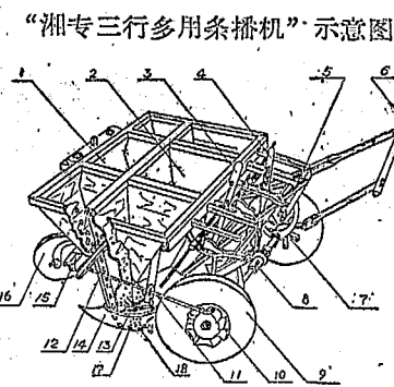
湘專三行多用小麥條播機
