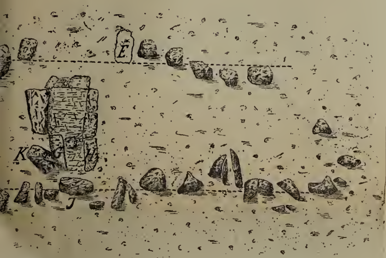
n unter Boden, G, H, J Tragsteine, K Deckstein vom Eingang.
