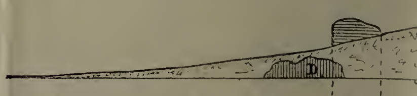
Abb. 7. Querschnitt durch Grab I beim G
