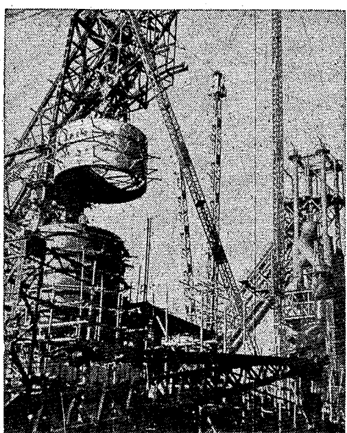
鞍鋼改造的第5座自動式高爐工程，正在安裝爐體和除塵器等設備。
