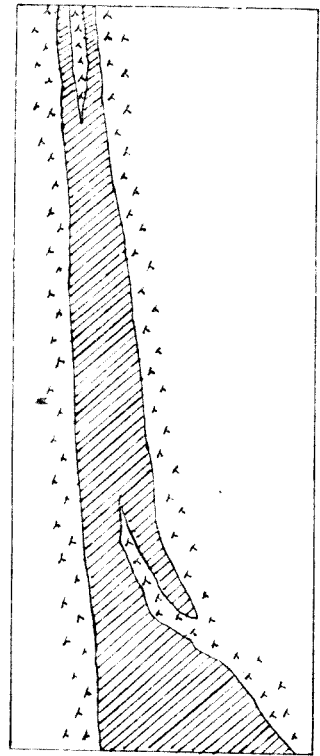
浙江湯溪縣 銀坑村鉛礦 剖面圖
