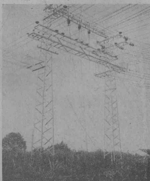
常州第一發電所33KV及2300V進出綫鋼塔
