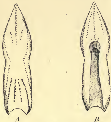
Fig. 64. C. parvidentata . A Pseudoconcha von unten, B von oben ( \frac{1}{2} ). Nach Pelsener.
