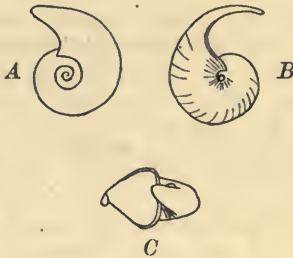
Fig. 8. L. inflata . A Schale von oben, B von unten, C von vorn. Nach Souleyet (15/2).
