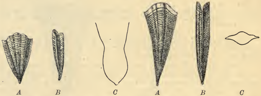
Fig. 26. C. recurva. A Schale von oben, B von rechts ( \frac{2}{3} ). Nach Orbigny. C Embryonalschale. Nach Pelseneer (vergr.?).
