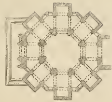
4. S. Maria della Salute in Venedig, Grundriss. (Nach Gurhle.)
