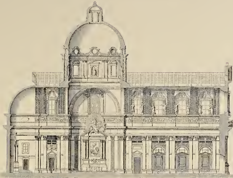
1. Il Gesù in Rom, Längsschnitt (vgl. Taf. 1).
