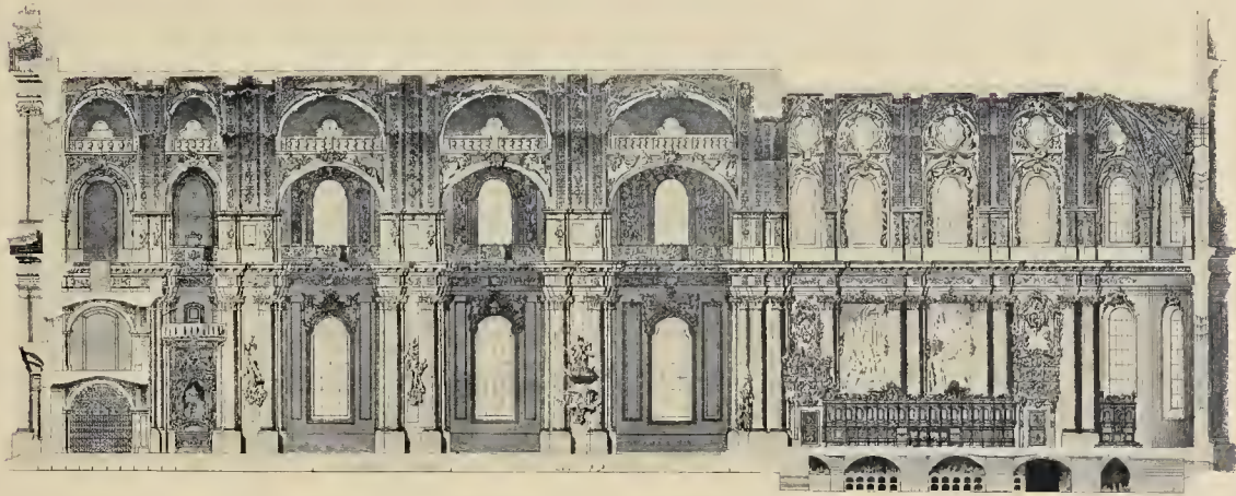
4. Kirche zu Fürstenfeld in Oberbaiern, 1718—1731, Längsschnitt.
