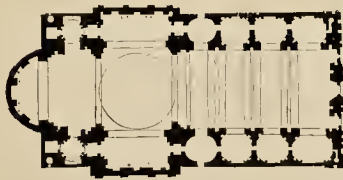
2. St. Petrus in Rom, Grundriss; von Vignola, 1568.
