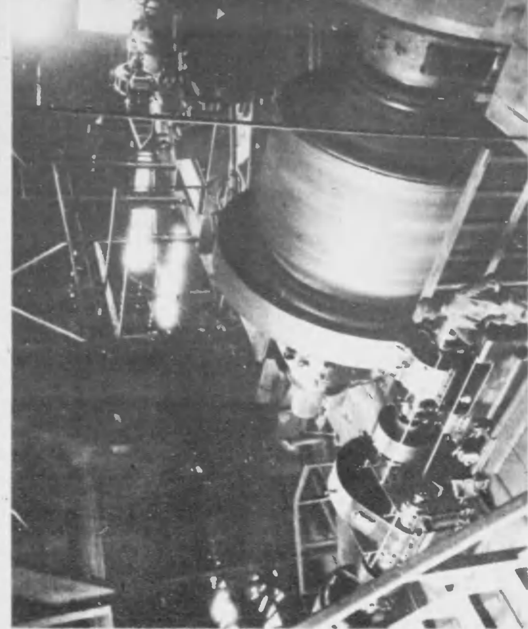
〇 鑛山より採られた鑛石は、選別機にかけて粉砕されるのもである (豊石鑛山)
