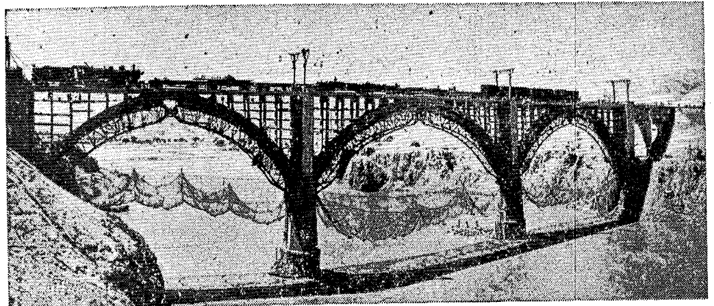
5月29日，第一列滿載鋼材、枕木的火車通過了包蘭鐵路黃河大拱橋。（新華社記者胡越攝）
