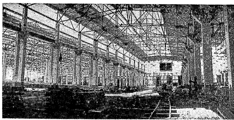
建設第一拖拉機製造廠的工人，只用38個工作日，就完成了拖拉機心機——發動機的製造工廠的廠房建築工程，工程質量完全合乎標準。
