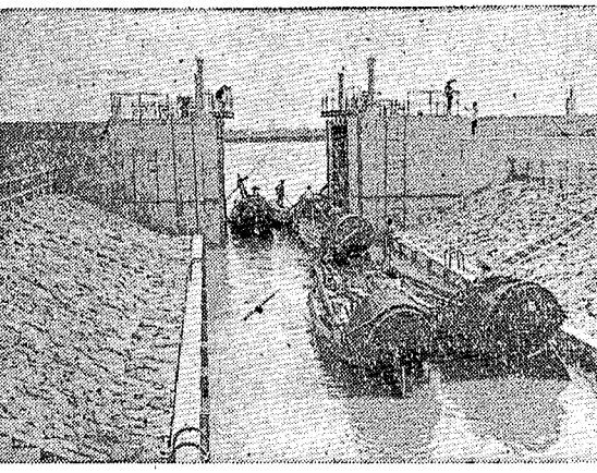
黃茅洲船閘建成後航運便利了 大通湖黃茅洲船閘建成後，每天都有上百艘船隻駛過黃茅洲船閘。船閘的建成，不但在水汛期可以通航，就是在洪水期間也可通航。(韓復祥攝)
