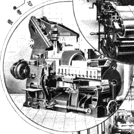
穿線訂書機
