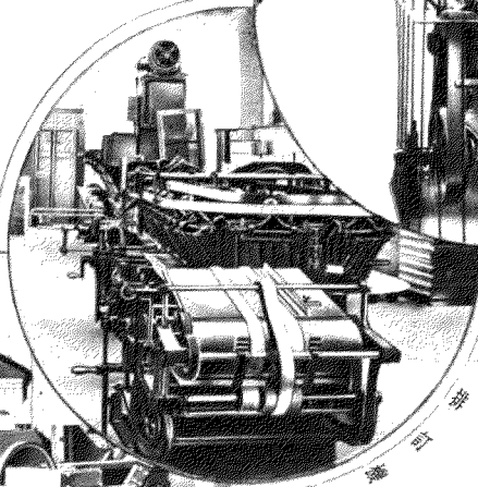
輪轉印機
