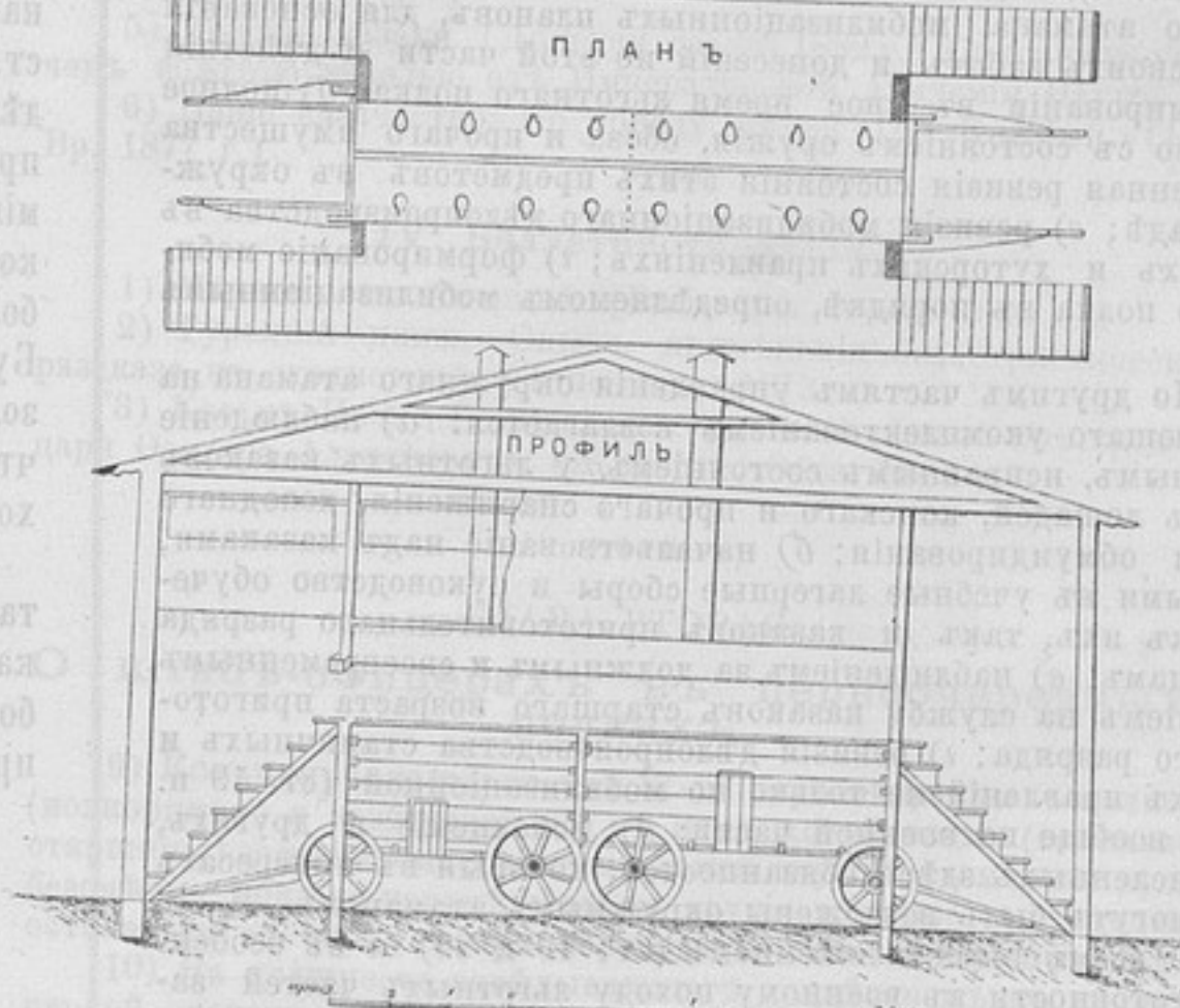
ПРОЕКТЪ ОТХОЖАГО МѢСТА НА БАТАЛІОНЪ (ВЫВОЗНОЙ СИСТЕМЫ)
