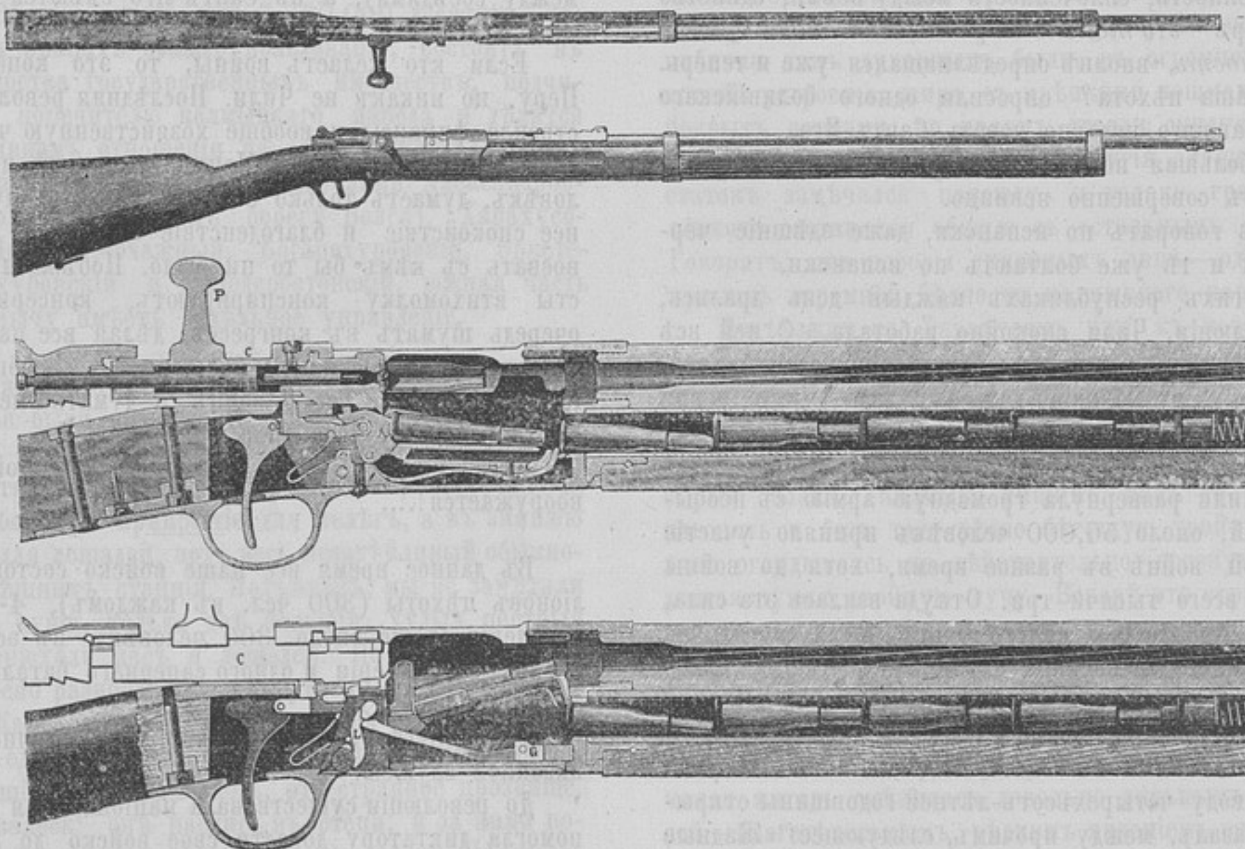
Французское 3-хъ линейное ружье Лебеля.
