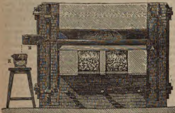
Фиг. 2. Заводское получение натрія по способу Девилля. АБ—железная трубка со смѣсью соды, угля и мѣла; В—холодильникъ Дони и Мареска; К—приемникъ съ нефтью.
