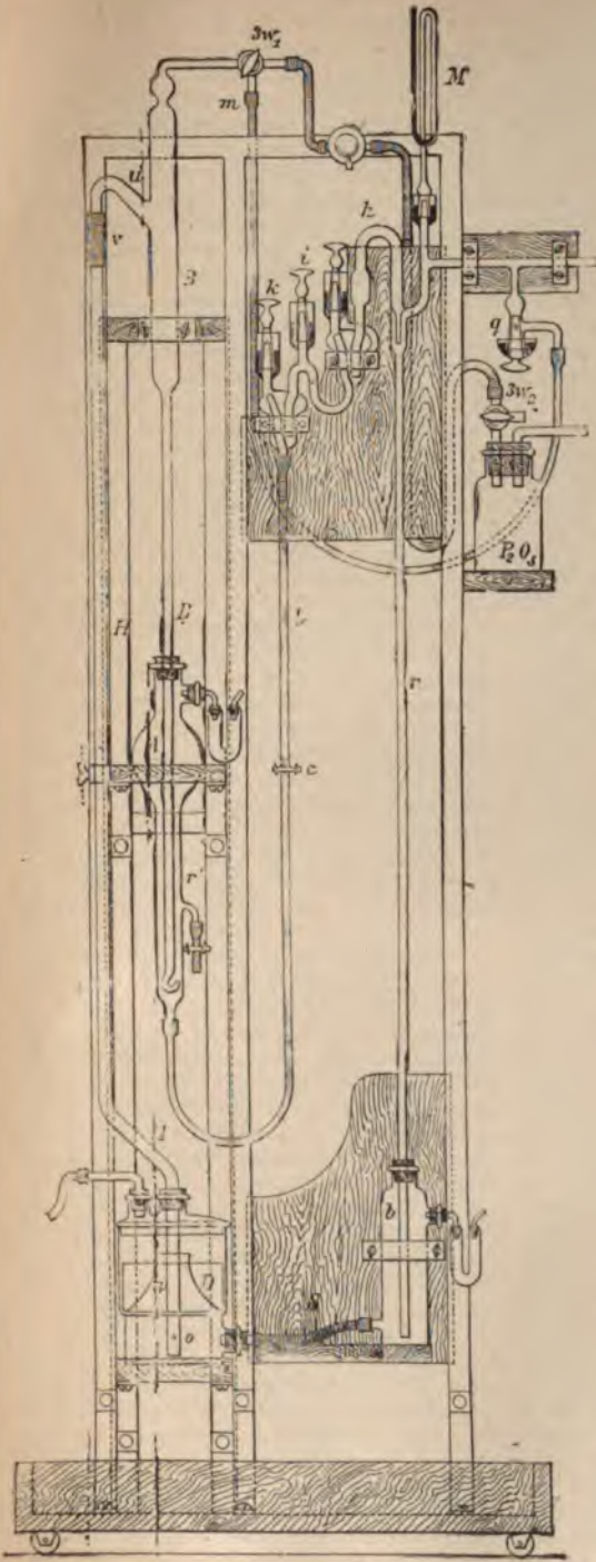
15. Ртутный воздушный П. Кальбауш.
