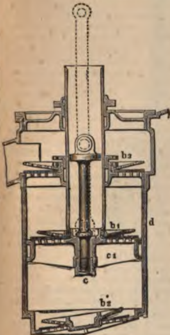
7. Воздушный насос Ватта
