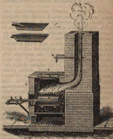
Фиг. 1. Полученіе калия, именно въ желѣзномъ сосудѣ А, въ которомъ смѣсь поташа, угля и мѣла. С — термометръ Дюппи и Марска. Вверху онъ же изображенъ въ разобранномъ видѣ.
