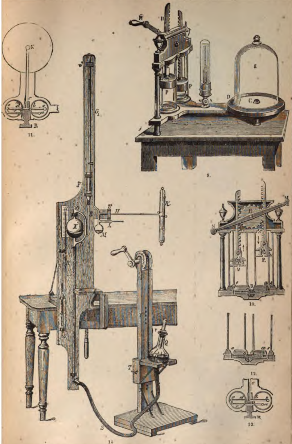
Фиг. 9—13. Двухцилиндровый воздушный насос. 14. Ртутный воздушный насос Бессель-Гагена.
