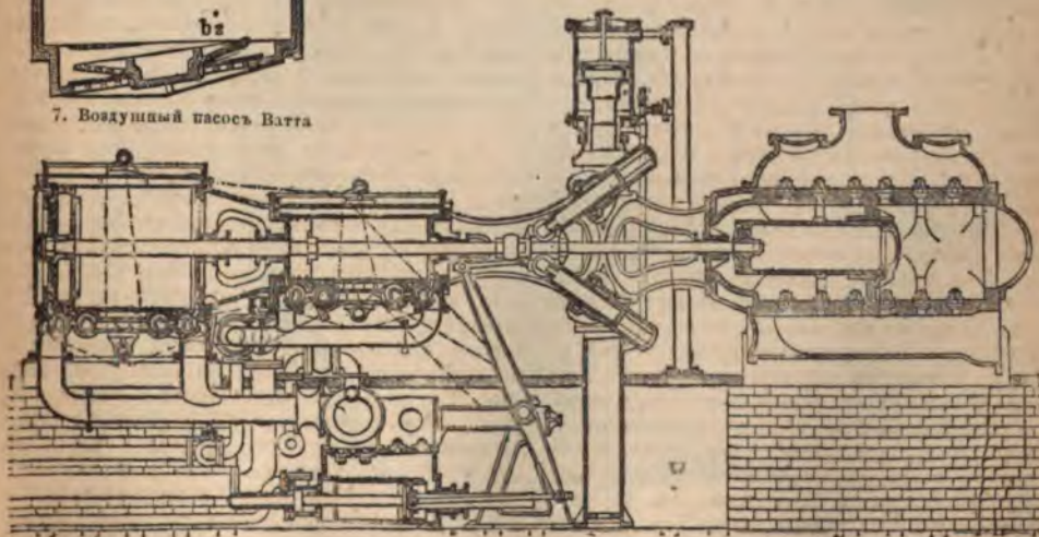
8. Насос Вортингтона.
