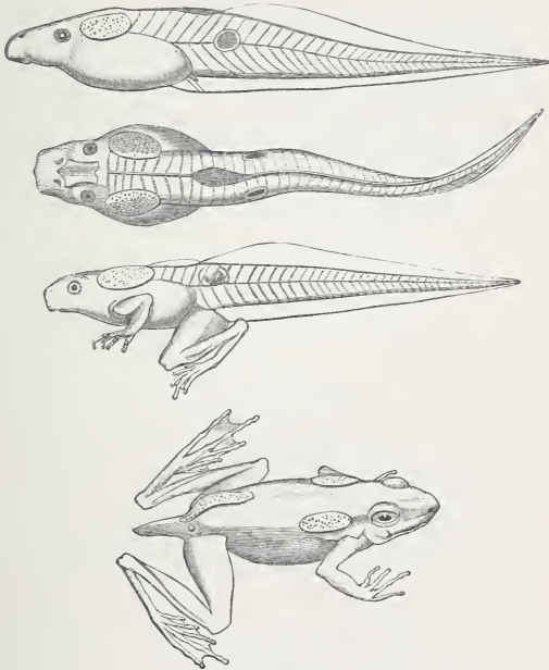
Rana alticola. Larvæ.
