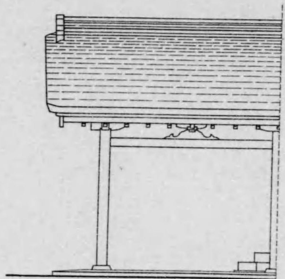
側面
