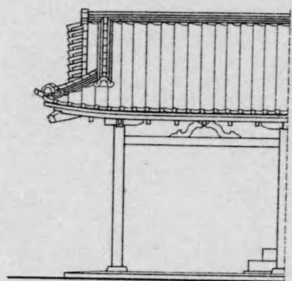
側面
