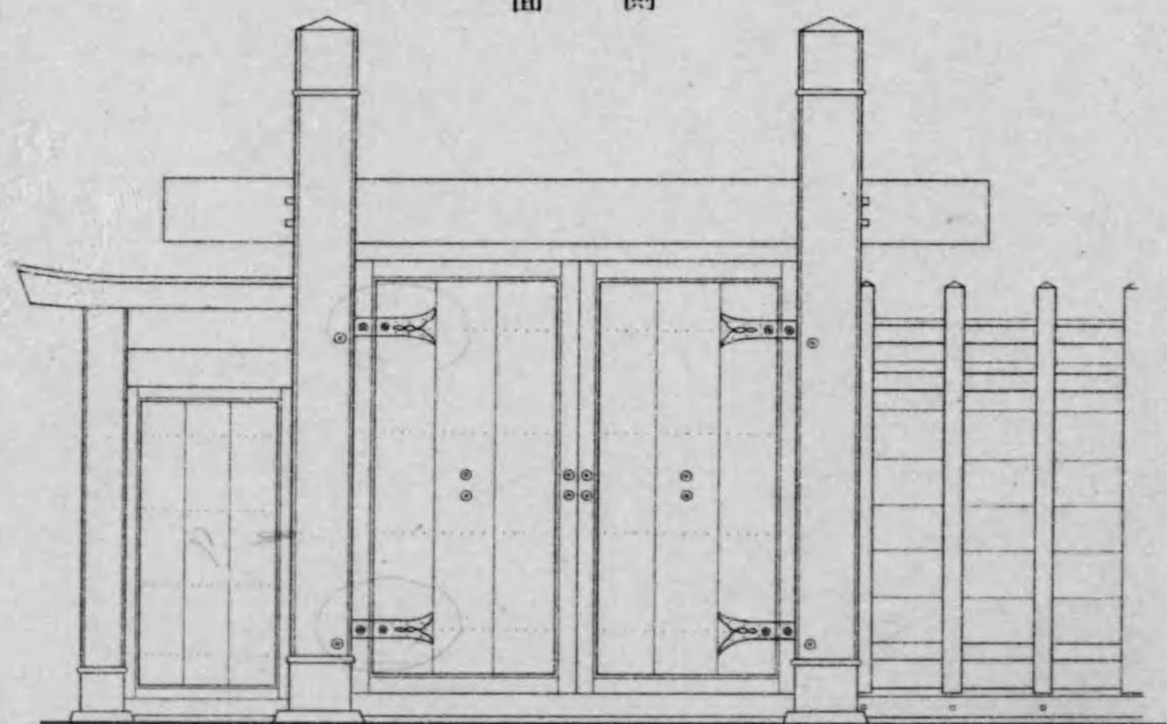
正面
