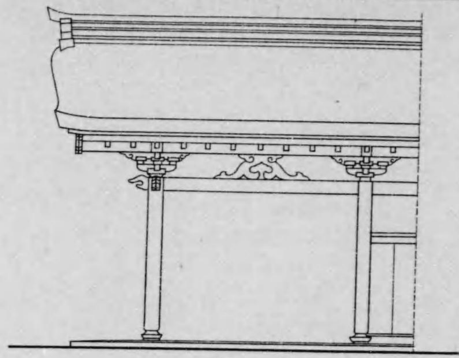
側面
