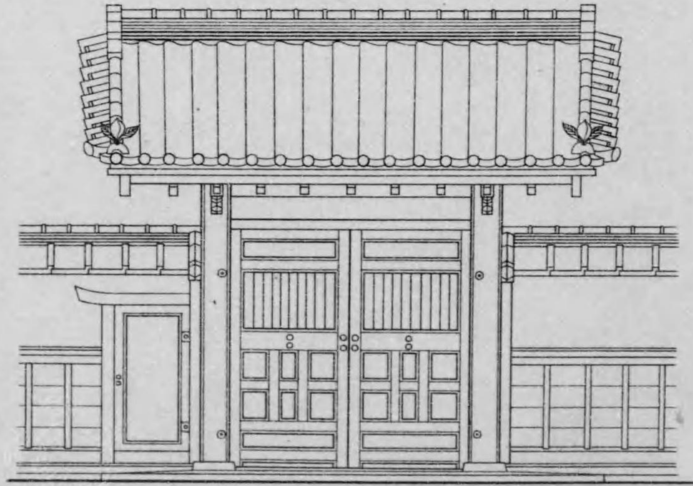
面正
