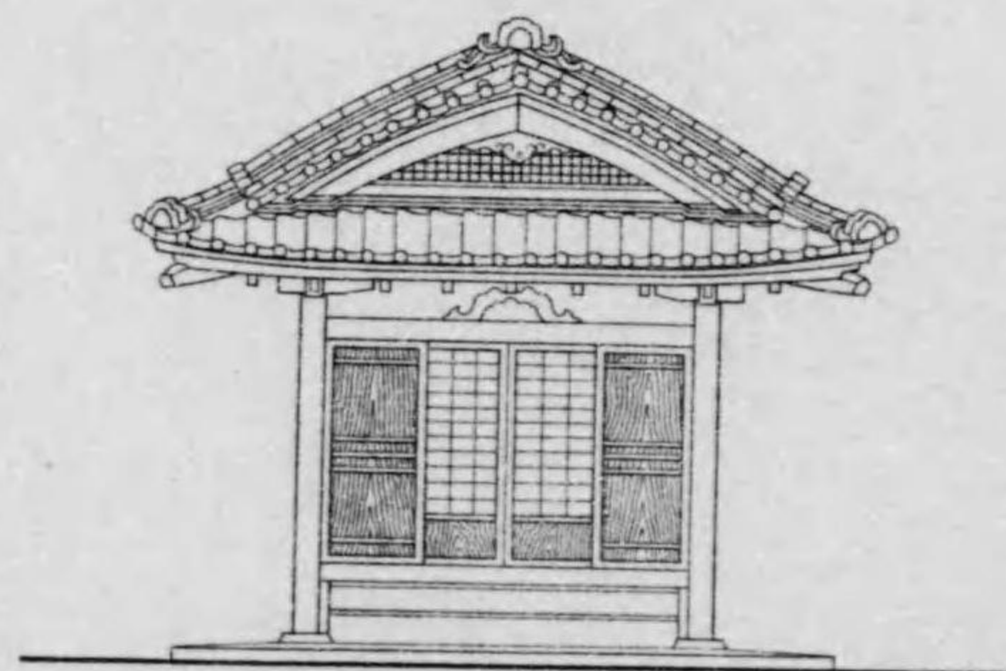
正面
