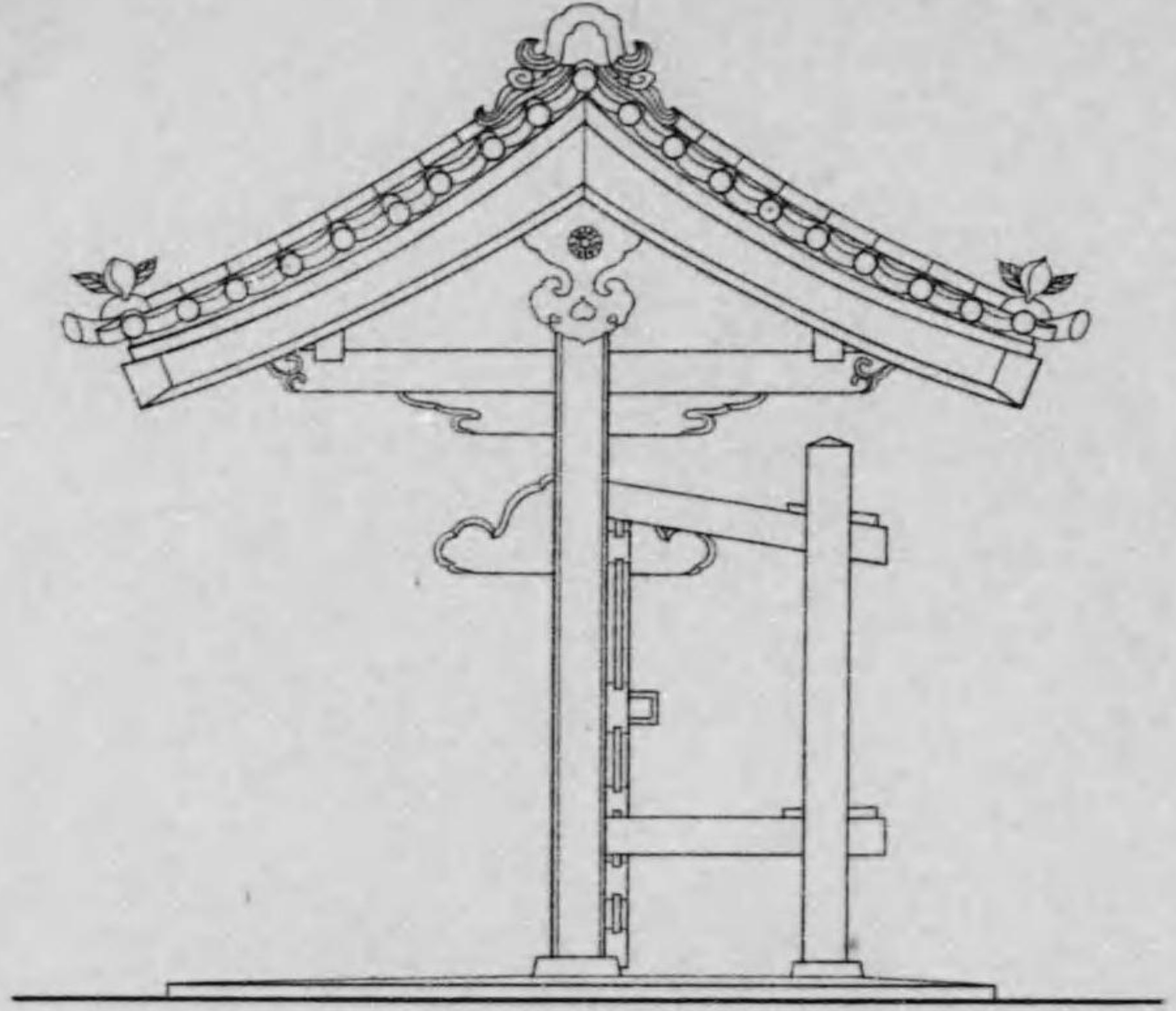
面側
