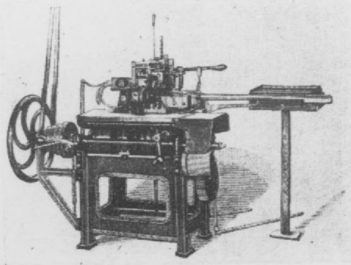
中國自製新式鑄字機
