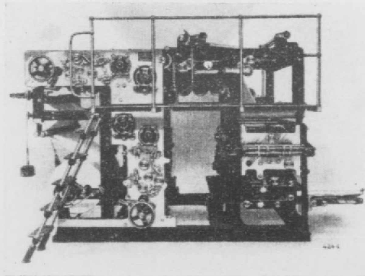
機報印轉運式高國美
