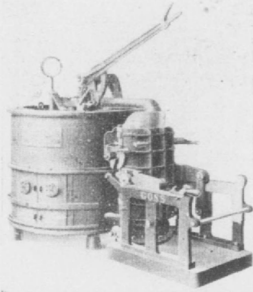
美國單邦浦烘鉛版機
