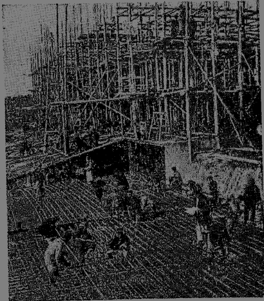
▲ 蘇家壩抽水閘是治湖工程中最大的建閘工程，參加建閘的數千工人正在緊張勞動。
