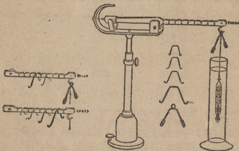
圖10. 莫兒氏天平
