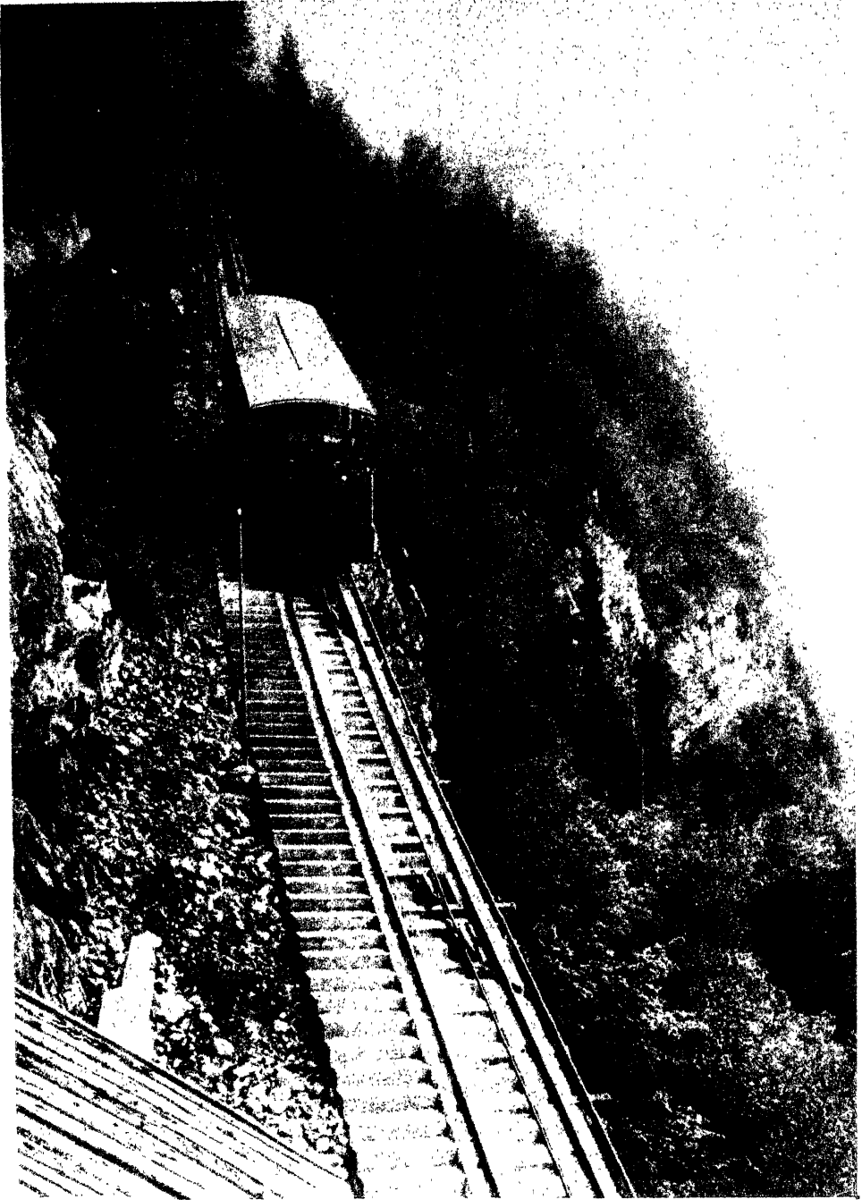
برگستانك فولی كولر ریلوی (خط آهن كوهی)
