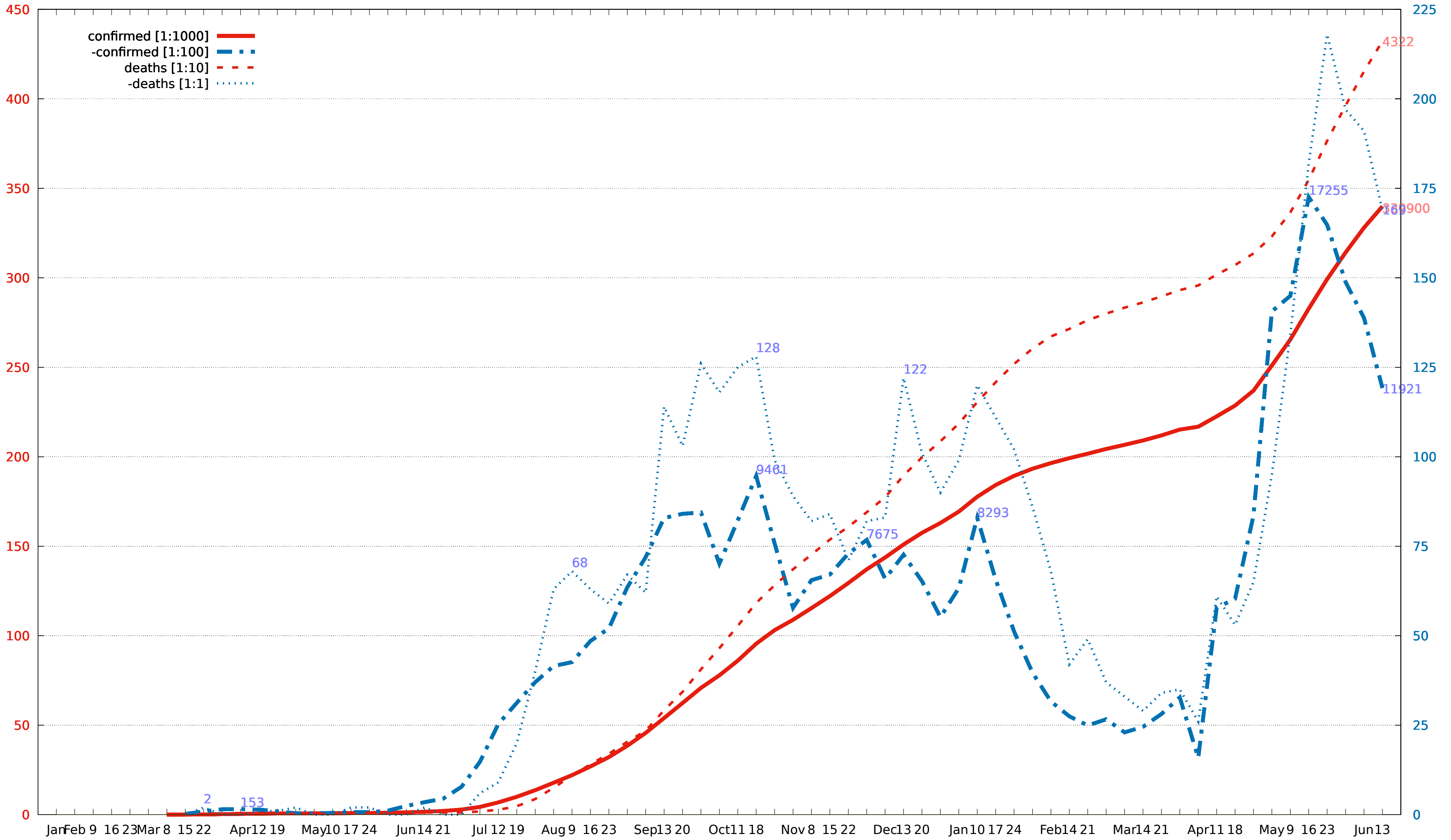
Costa_Rica
