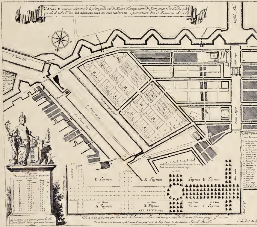
PLAN VAN AANLEG DER PLANTAGE, 1682 Gravure door B. Stoopendae
