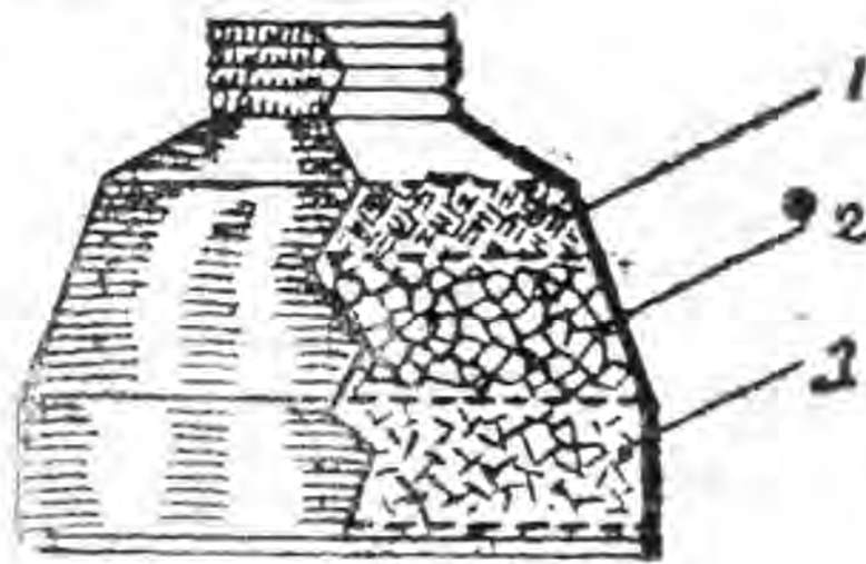
二十三圖 濾毒罐的剖解圖
