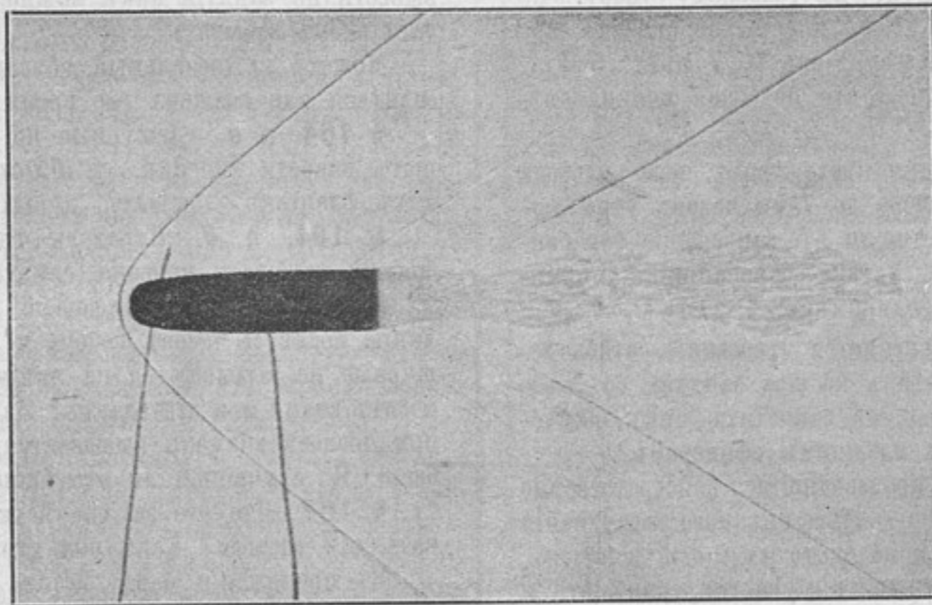
Фотографическій снимокъ съ летящей пули системы Ли-Энфильда, показывающій воздушныя волны, образующіяся впереди снаряда, и пустоту, остающуюся за нимъ, которая постепенно заполняется воздухомъ.
