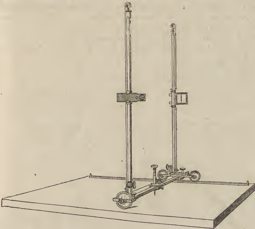
Diagraphe à deux montants.
