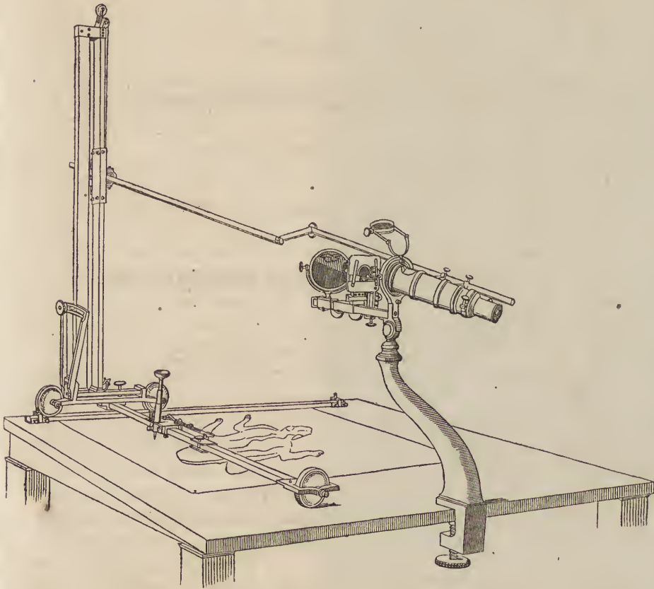
Diagraphe à microscope.
