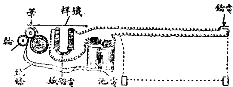
示電報機的裝置
