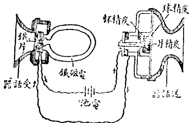
示 電 話 機 的 裝 置
