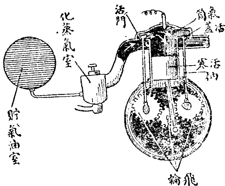
機 動 發 油 氣
