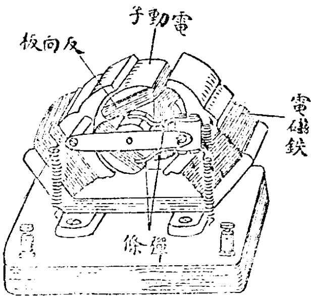
機 動 電
