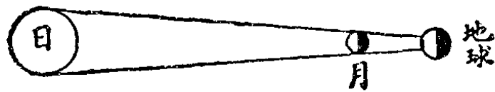
食 日
