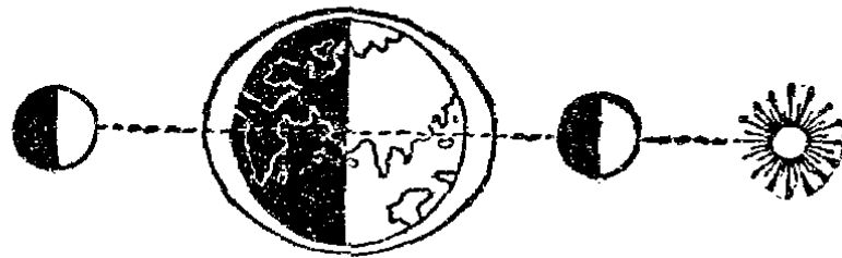
大潮或汐大
