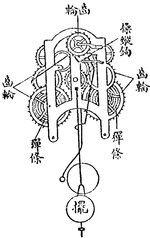
時鐘的內部
