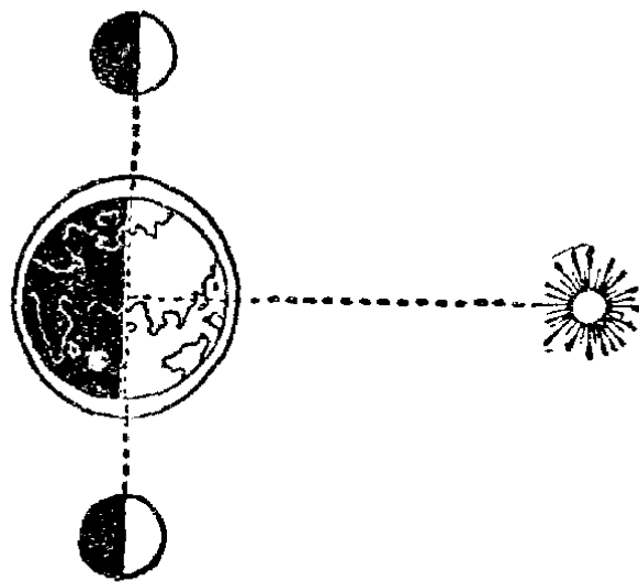
小潮或汐小
