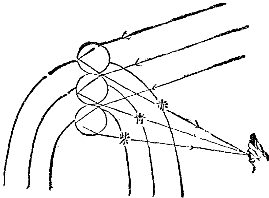
虹 的 成 因
