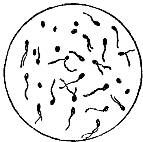
菌 細
