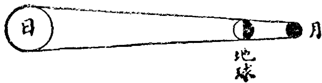
食 月
