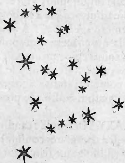
NEBVLOSA ORIONIS.
