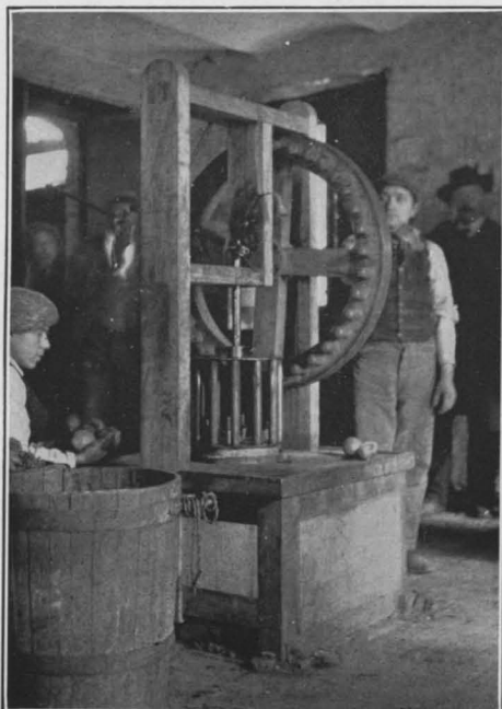
FIG. 2.—LEMON-OIL MACHINE, REGGIO, CALABRIA.
