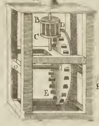
Fig. 12. Grinding
