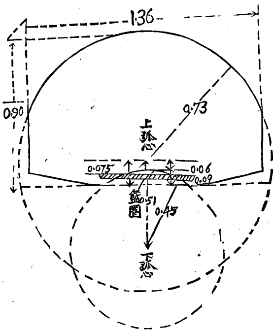
扇形遮板圖
