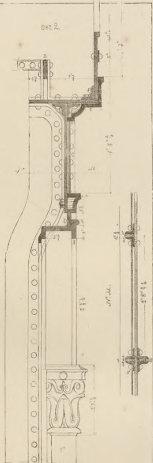
Fig. 3. PLAN DE LA COLONNE
