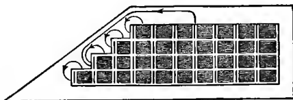
Fig. 39. Scheme of myomeres in an oblique section (Rosenthal).
