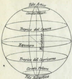
Circoli della Sfera
