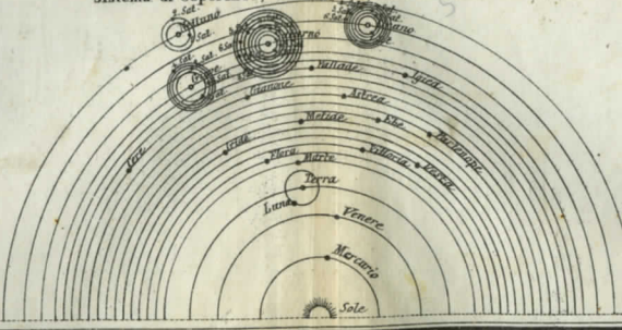
Sistema di Copernico, Galileo, ecc. ossia Sistema attuale.
