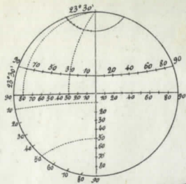
Divisione dei Circoli
