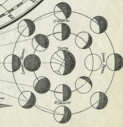
Fasi della Luna
