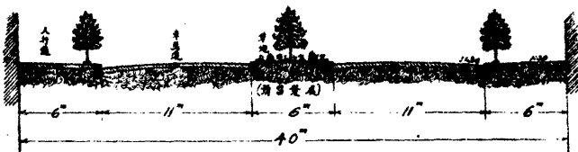
40' 馬路標準 (二等馬路)
