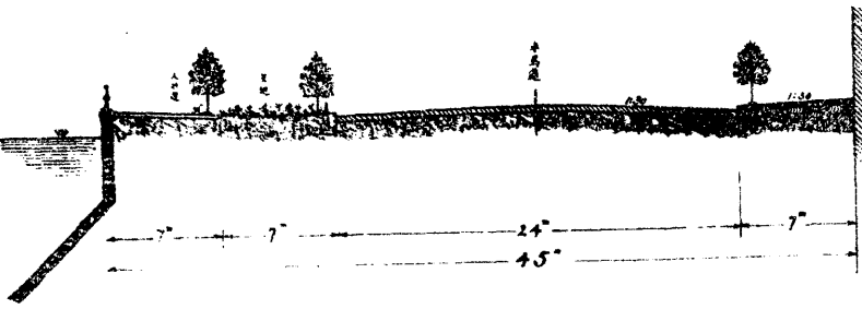
沿江馬路 (一等馬路)
