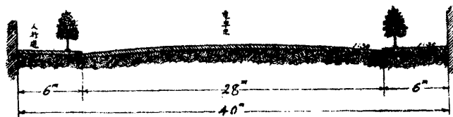
40' 馬路標準 (二等馬路)
