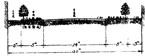
150' 馬路標準 (三等馬路)
