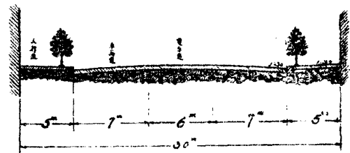
120' 馬路標準 (三等馬路)
