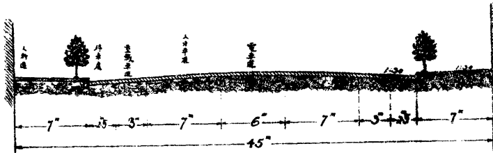
45' 馬路標準 (一等馬路)
