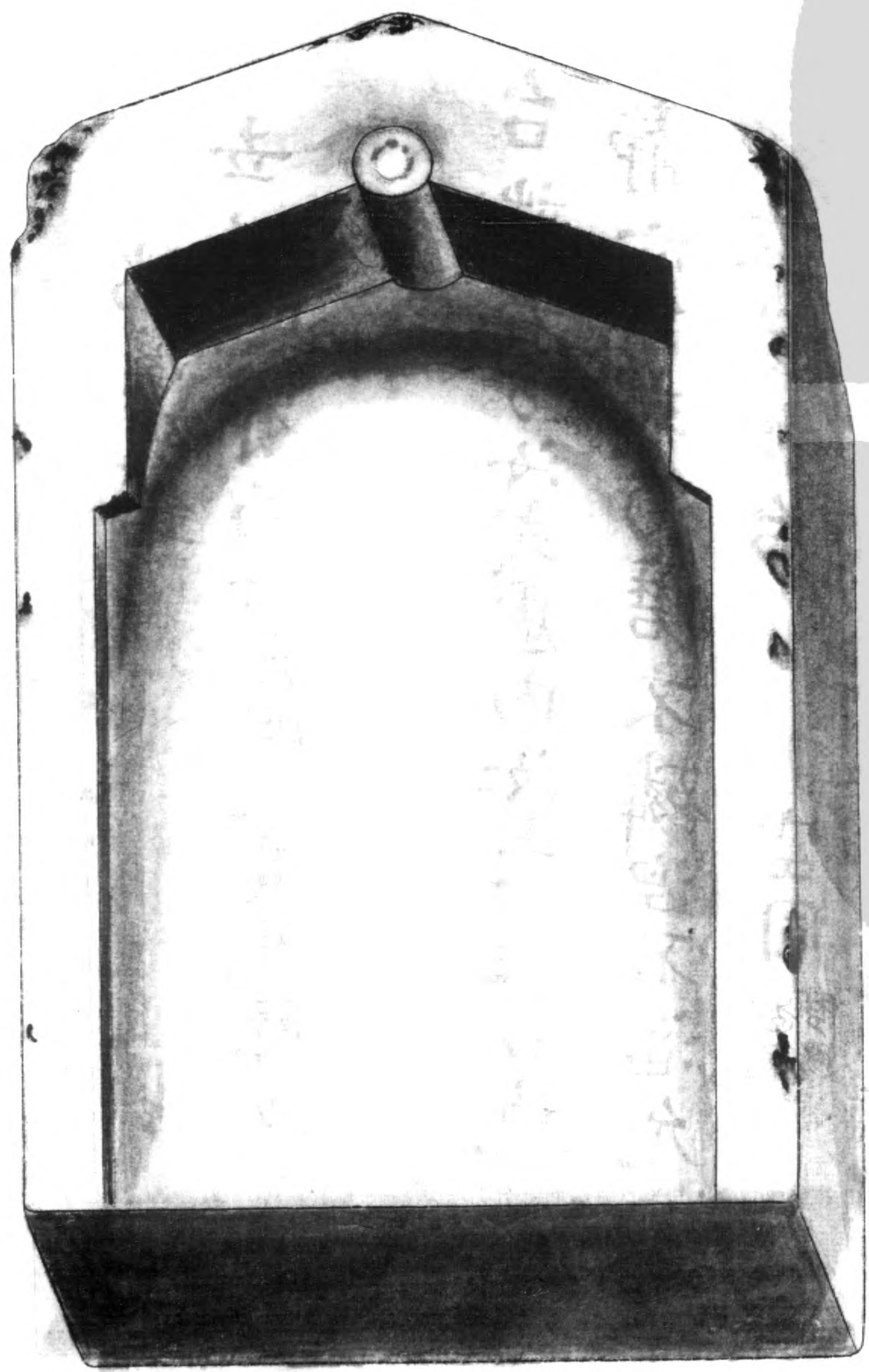
明李夢陽端石圭硯正面圖 繪圖十分之五
