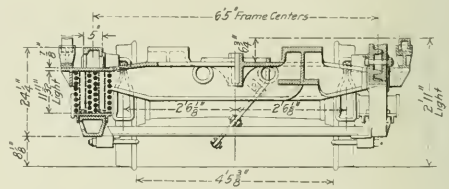
Section A-A-A-A
