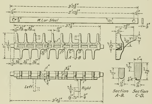
Fig. 2—Finger Grate Bar.
