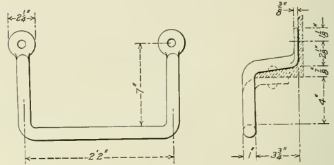
Fig. 6—Cylinder Lever Guide.
