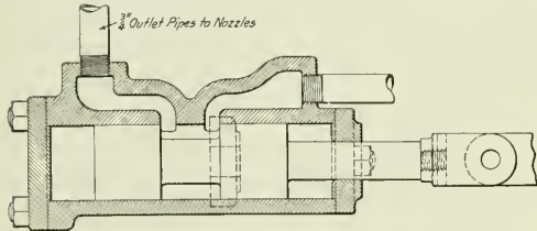
Section A-B
