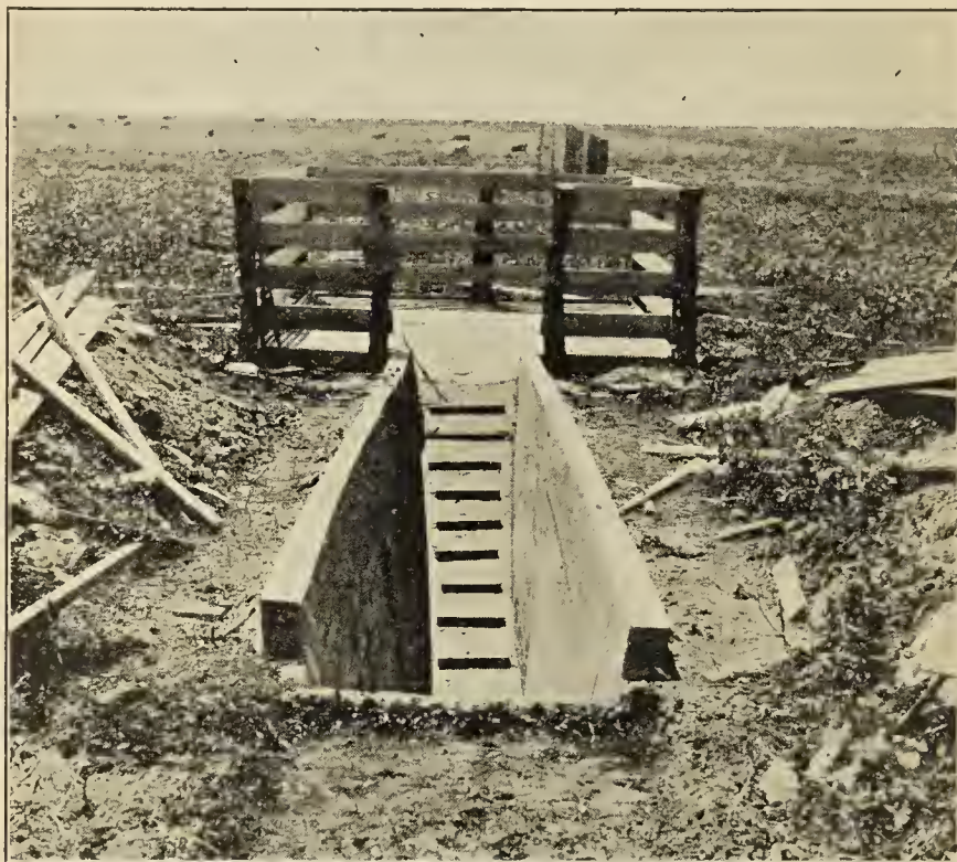
Este grabado muestra como se construye el tanque o zanja.
