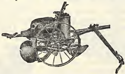
The 100% Potato Planter
