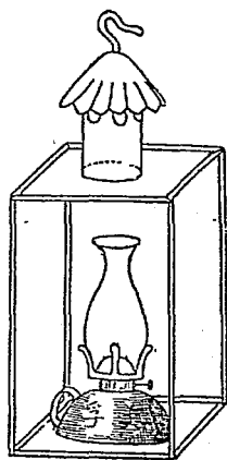
第三十三圖 誘蛾燈的避風裝置
