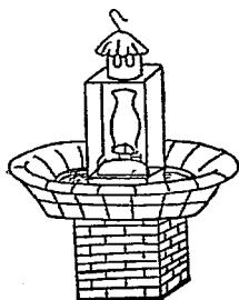
誘蛾燈的磚臺安放裝置
