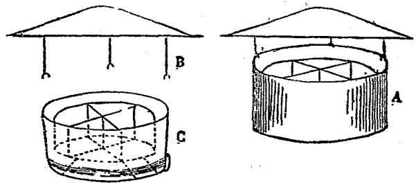
第四式寄生蜂保護器
