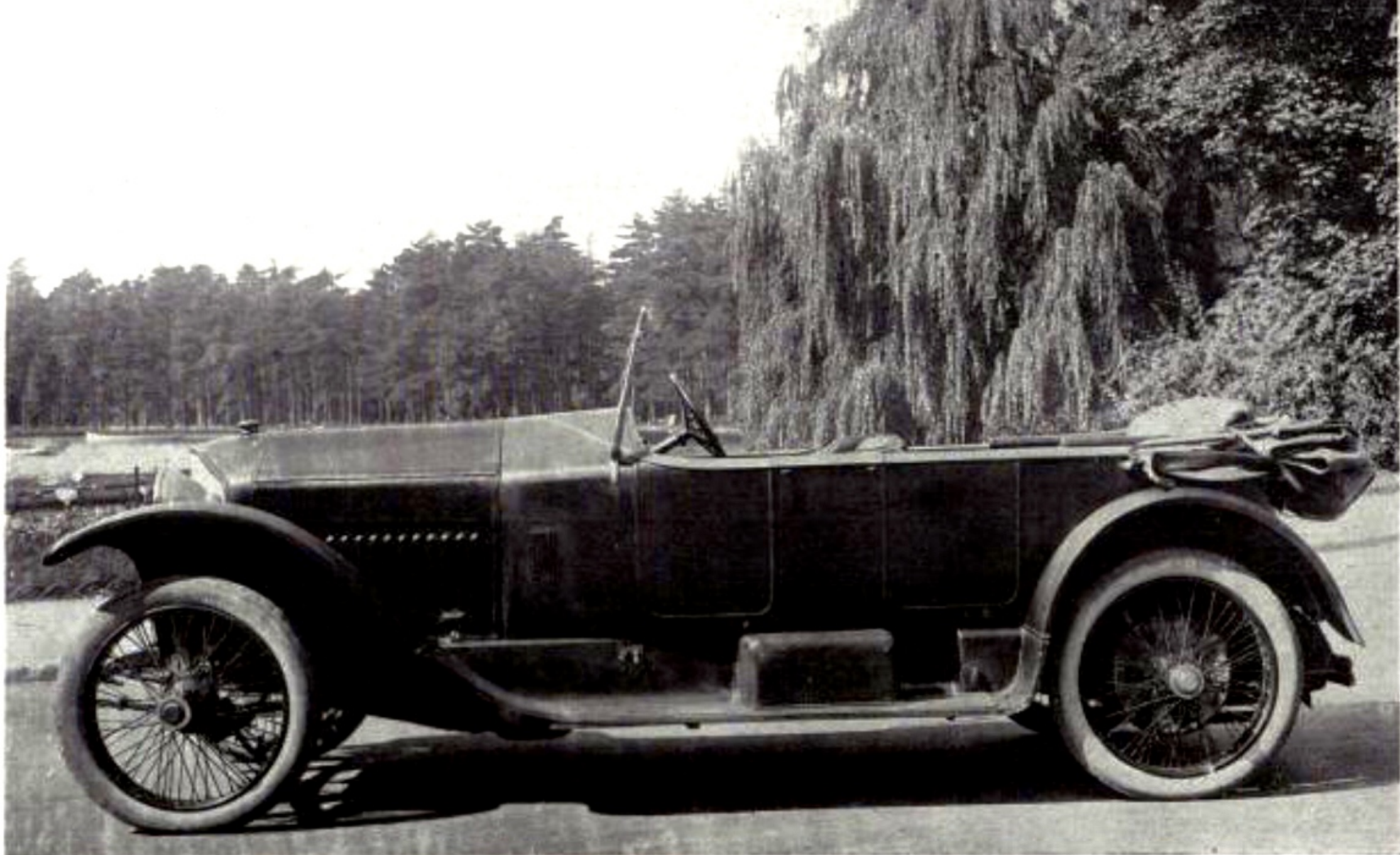
PICCARD PICTET. — LE TORPÉDO QUATRE PLACES. REMARQUEZ QUE DANS LE TORPÉDO MODERNE, LES DOSSIERS DES BANQUETTES SONT RAMENÉS A LA HAUTEUR DES PANNEAUX LATÉRAUX. C'EST EXACTEMENT LE CONTRAIRE DE CE QUI SE FAISAIT DU TEMPS DES « TULIPES » ET DES CARROSSERIES « ROI DES BELGES ».
