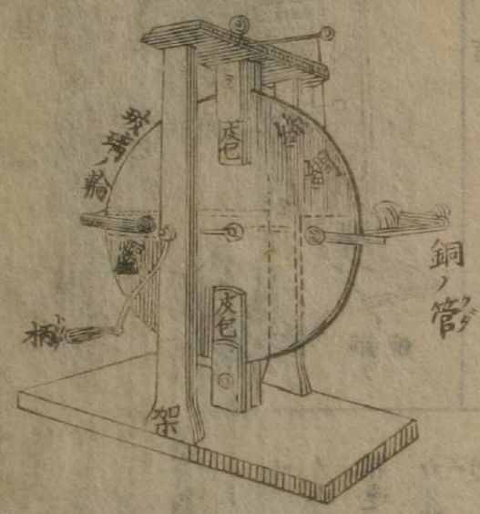
電機器ノ圖
