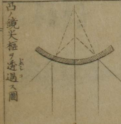
外景ノ凹鏡ニルノ圖
