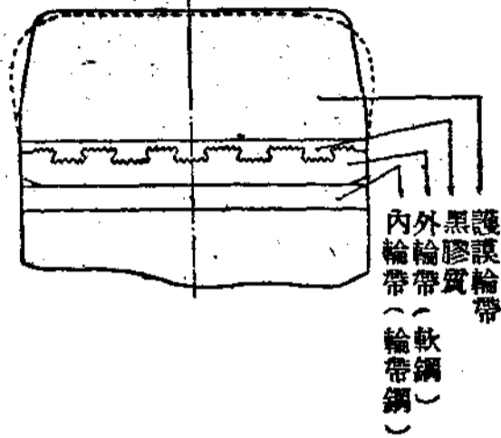
附圖第四 輪帶一般形狀之斷面（其一）
