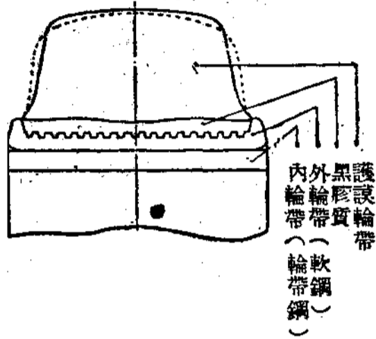
輪帶一般形狀之斷面 (其二)
