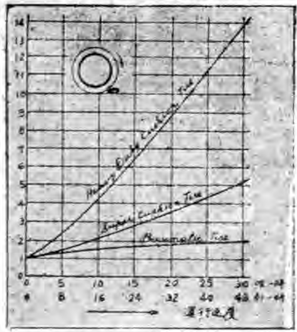
附圖第三各種輪帶緩衝度曲線
