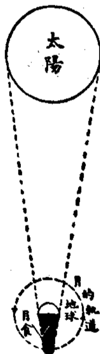
月食圖
